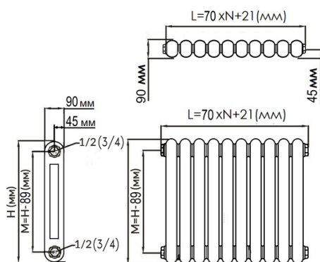
Боковое подключение
