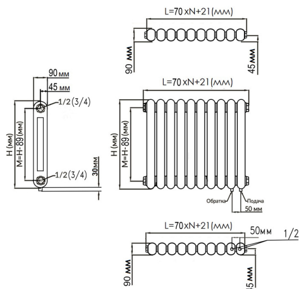
Нижнее подключение
