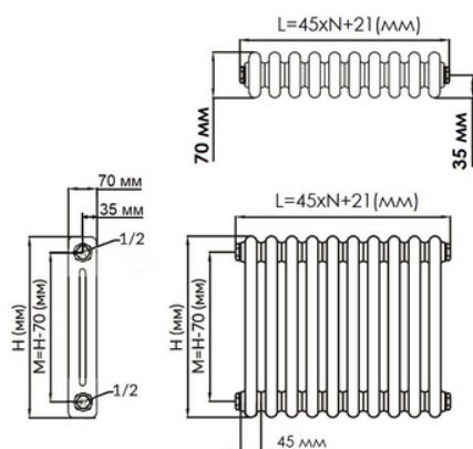
Боковое подключение
