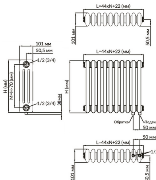
Нижнее подключение
