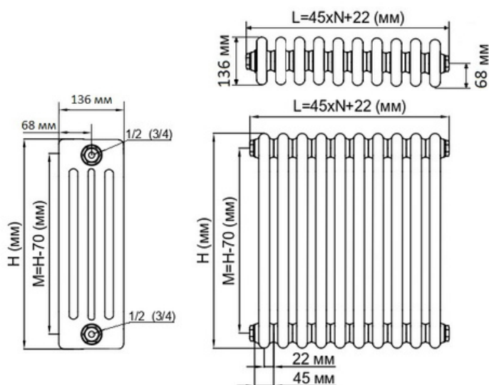
Боковое подключение
