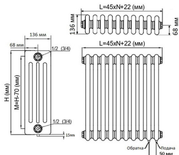
Нижнее подключение
