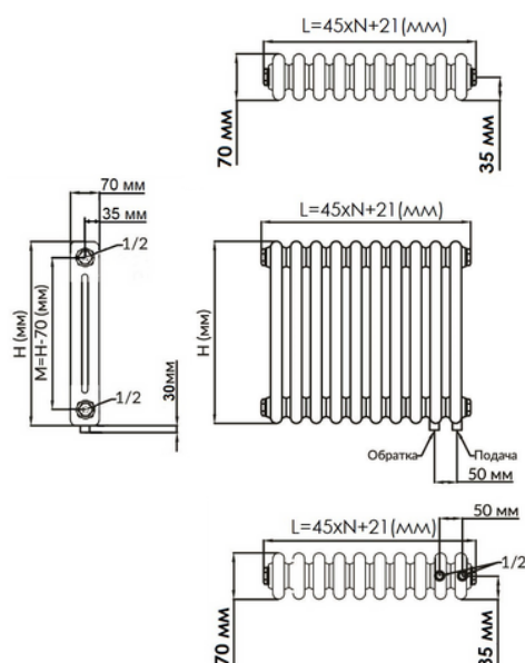
Нижнее подключение
