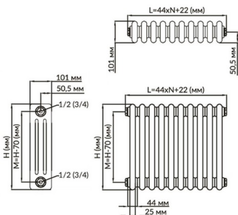
Боковое подключение
